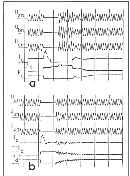
Fig. 7 Transientes Verhalten bei wiederkehrender Spannung
