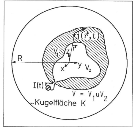
Fig. 1 Komplizierte Leiterstruktur
