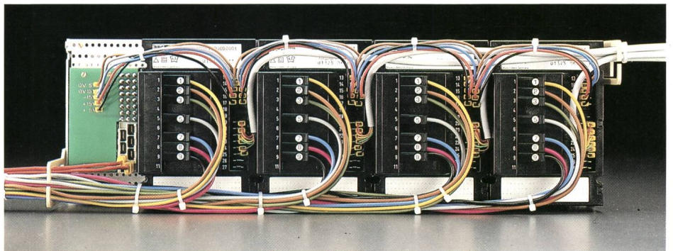
Rückansicht Baugruppenträger
