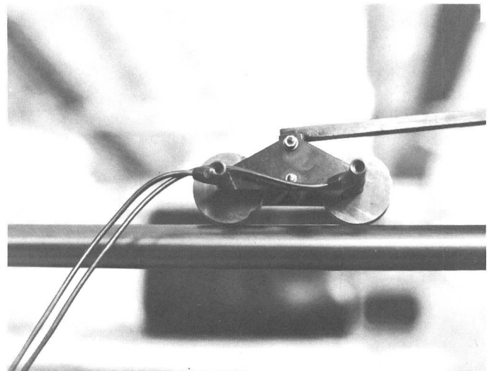
Fig. 1b Kabel und Abgriffrollen mit Messleitungen (s. auch Fig. 1a)
