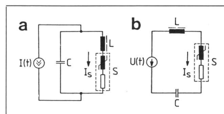
Fig. 2 Circuits de résonance RLC avec excitation périodique à impulsions
