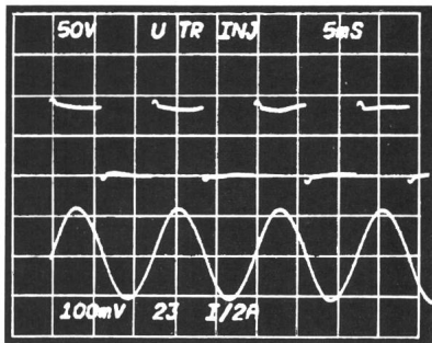
Fig. 5 Oscillogrammes de la tension injectée par le transformateur T_{r1} (en haut) et du courant de charge (en bas) dans le cas de la source de courant de la figure 4
