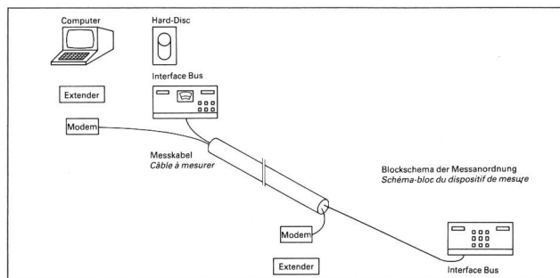
Über 20 000 Prüfwerte wurden am computergesteuerten Messplatz erfasst.
