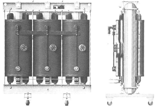
Giessharz-Transformatoren Glasfaser/Harz-Transformatoren
