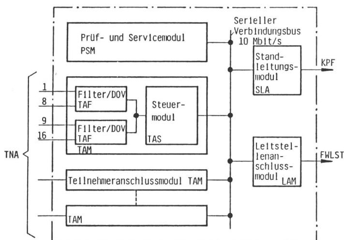
Fig. 5 Aufbau des Koppelfeldes TNA: Telemetrie-netz-abschluss KPF: Koppelfeld FWLST: Fernwirk-leitstelle
