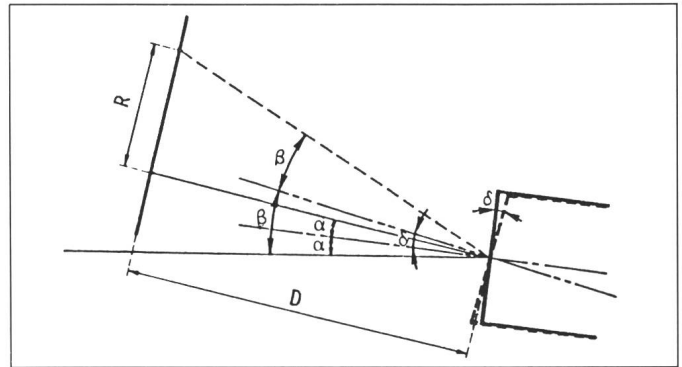
Fig. 8 Berechnung des Endflächenwinkels \delta = 1/2 \arctg(R/D)
