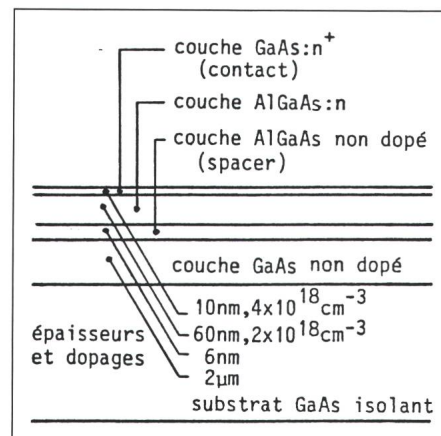
Fig. 10 Composition et épaisseurs typiques des couches épitaxiales MBE utilisées pour la réalisation des structures Tefget
