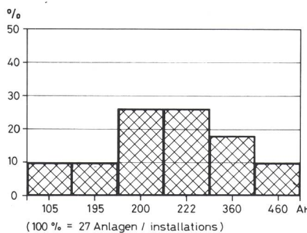
Fig. 6 Batterie-Kapazitäten, prozentuale Verteilung / Capacités des batteries, répartition en %
