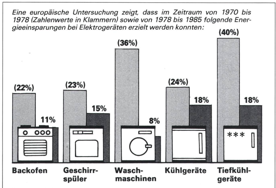
Fig. 2 Elektrizitätseinsparungen durch technische Verbesserungen von elektrischen Haushaltgeräten
