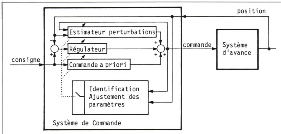
Figure 2 Schéma global du système de commande d'axe
