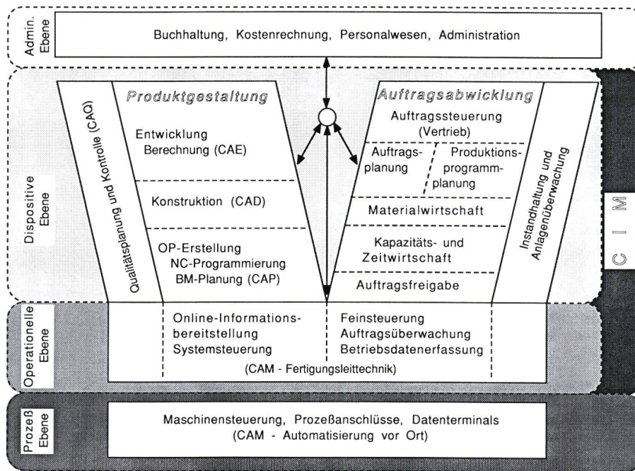
Figur 1 Systemarchitektur der verschiedenen EDV-Funktionen eines Betriebes.
