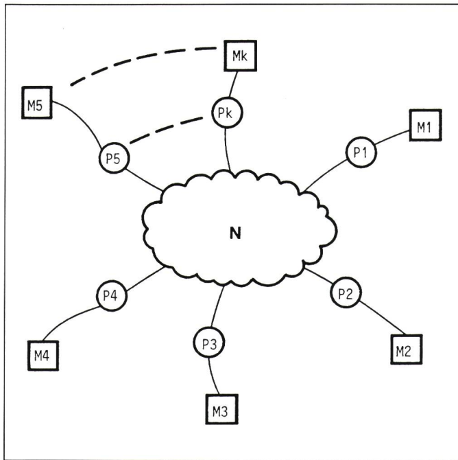
Figur 5 Verteiltes System
