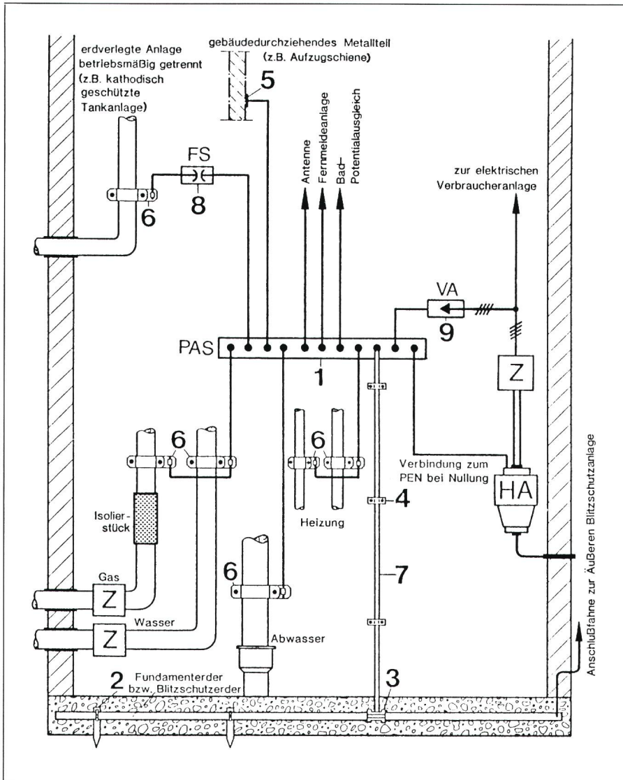
Figur 2 Potentialausgleich
