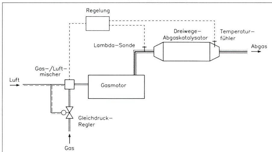
Figur 1 Dreiweg-Abgaskatalysator Prinzipischema
