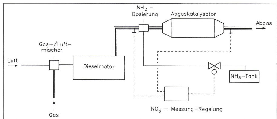
Figur 4 SCR-Abgaskatalysator Prinzipschema
