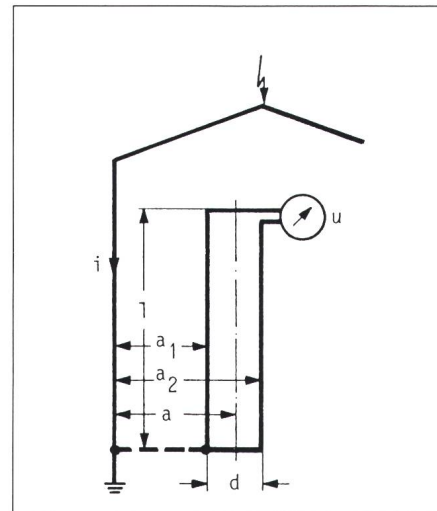
Figur 13 Induktionsspannung in einer Schleife
