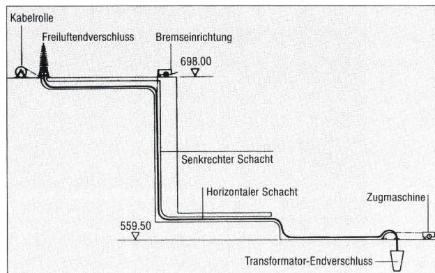
Übersichtsschema der Kabelanlage.
