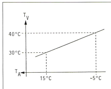
Figur 2 Heizgerade
