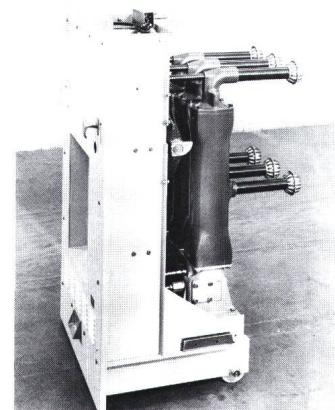
Figur 3 SF 6 -Leistungsschalter Typ HB (Selbstblasprinzip)
