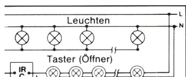
Infracontrol als Treppenlicht-Automat in Tasterschaltung:
