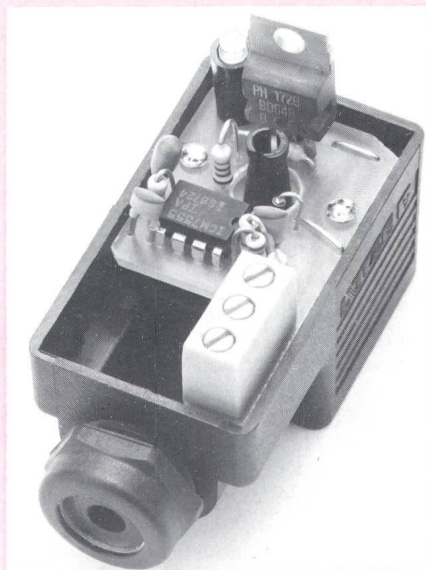
Gerätestecker Lütze-Variocontact
