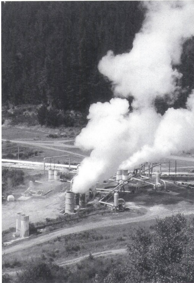
Bild 1 Geothermische Kraftwerke haben einen enormen Flächenbedarf. Wasser und Dampf aus dem Innern der Erde gelangen in kilometerlangen Pipelines vom geothermischen Feld zur Zentrale, die sich in der Nähe eines Flusses befinden muss.
