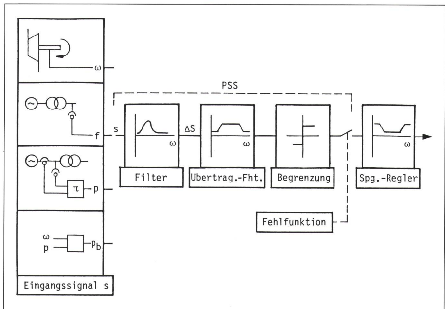
Bild 3 PSS-Grundschemata \omega Drehzahl f Frequenz p Wirkleistung P_b Beschleunigungsleistung
