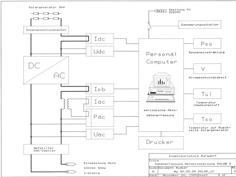
Bild 1 Blockschema der 3-kW-Photovoltaikanlage SOLAB 3.
