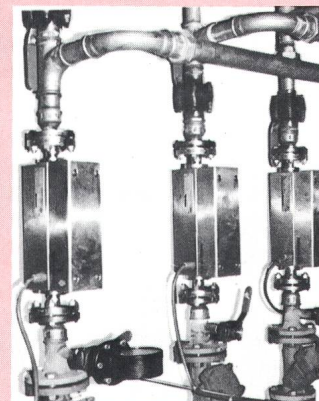
«m-point» Durchflussmessung
