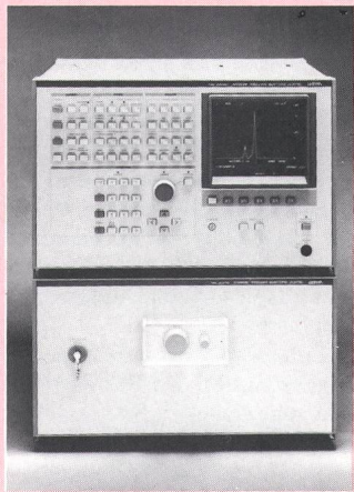
Optischer Spektralanalysator
