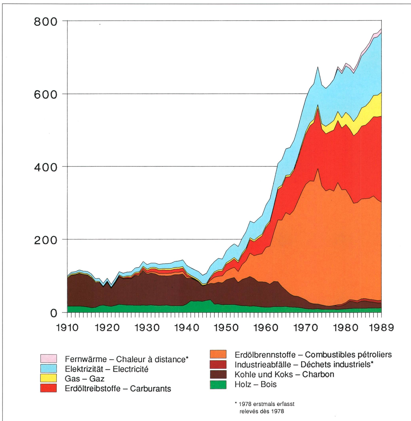
Fig. 1 Endenergieverbrauch 1910–1989 nach Energieträgern (in 1000 TJ) Consommation finale 1910–1989 selon les agents énergétiques (en 1000 TJ)
