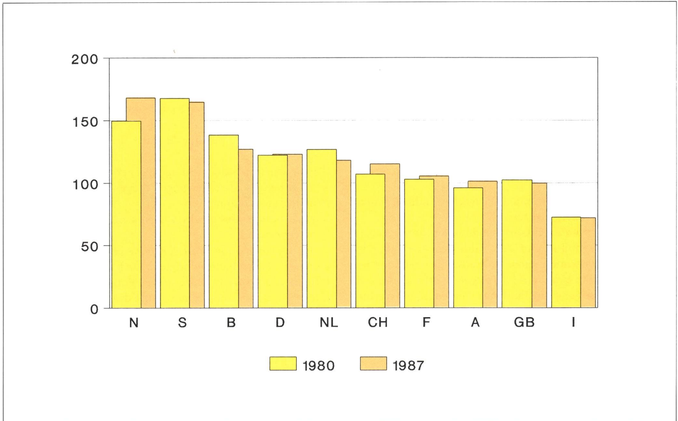
Fig. 3 Energieverbrauch pro Kopf in 1000 MJ Consommation d'énergie par habitant en 1000 MJ
