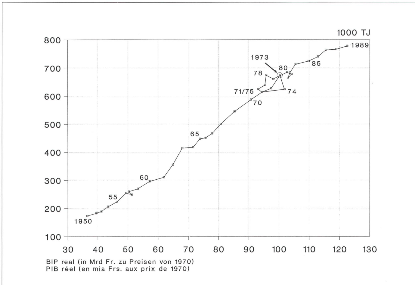
Fig. 9 Zusammenhang zwischen Endenergieverbrauch und wirtschaftliche Entwicklung Relation entre la consommation finale et l'évolution économique
