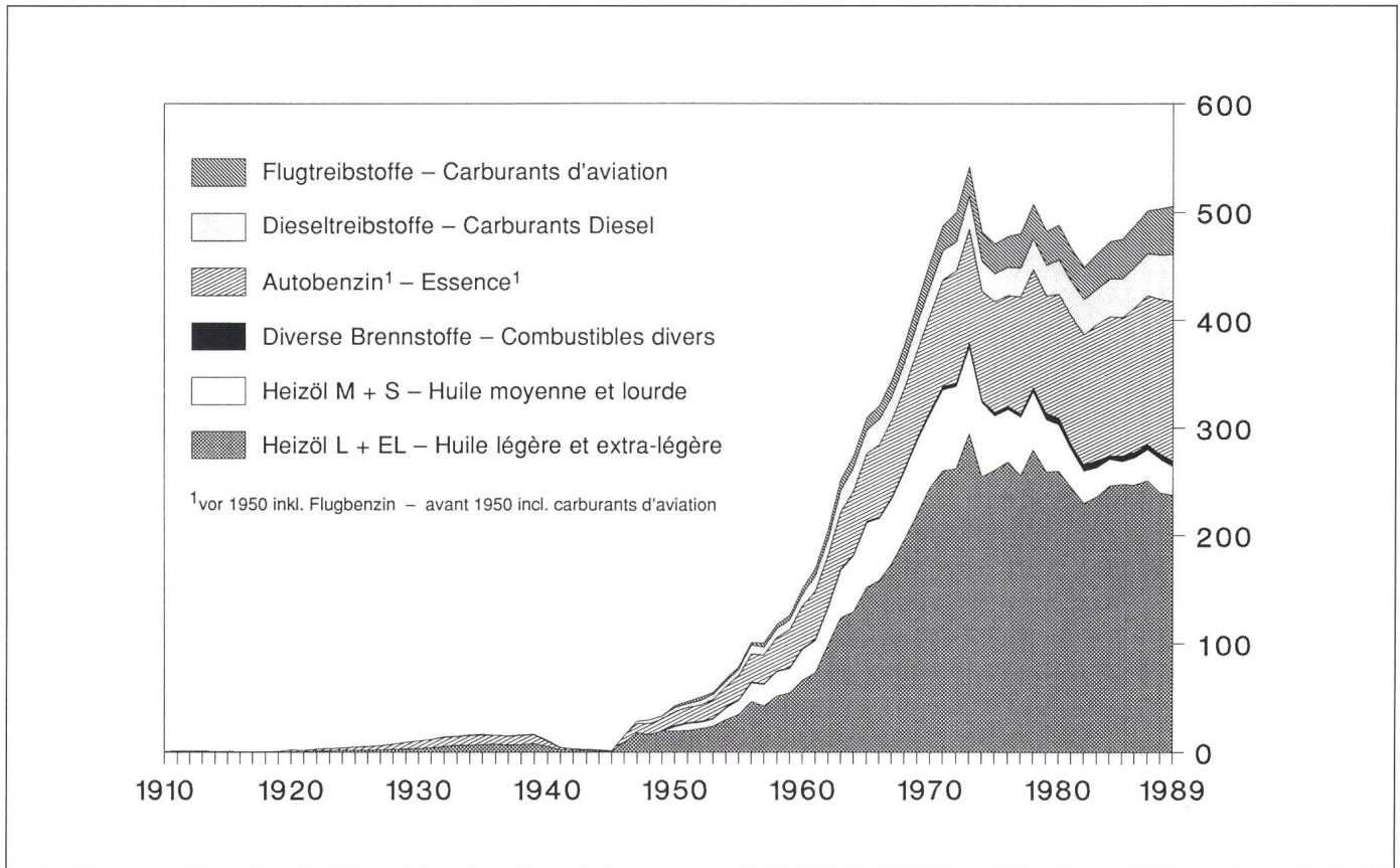
Fig. 7 Entwicklung des Endverbrauchs an Erdölprodukten (in 1000 TJ) Evolution de la consommation finale des produits pétroliers (en 1000 TJ)
