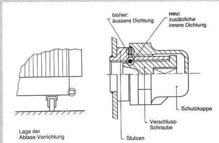
Neue Öl-Ablassvorrichtung DIN 42551 Trafosuisse
