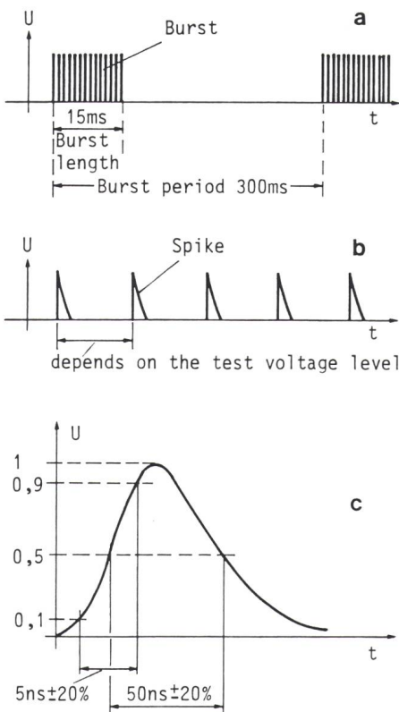
Bild 5 IEC-Prüf-Impuls für schnelle Transienten
