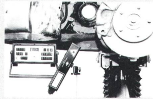
Torsions-Schwingungsmesser 2523
