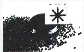
Filière pour fil polymer
