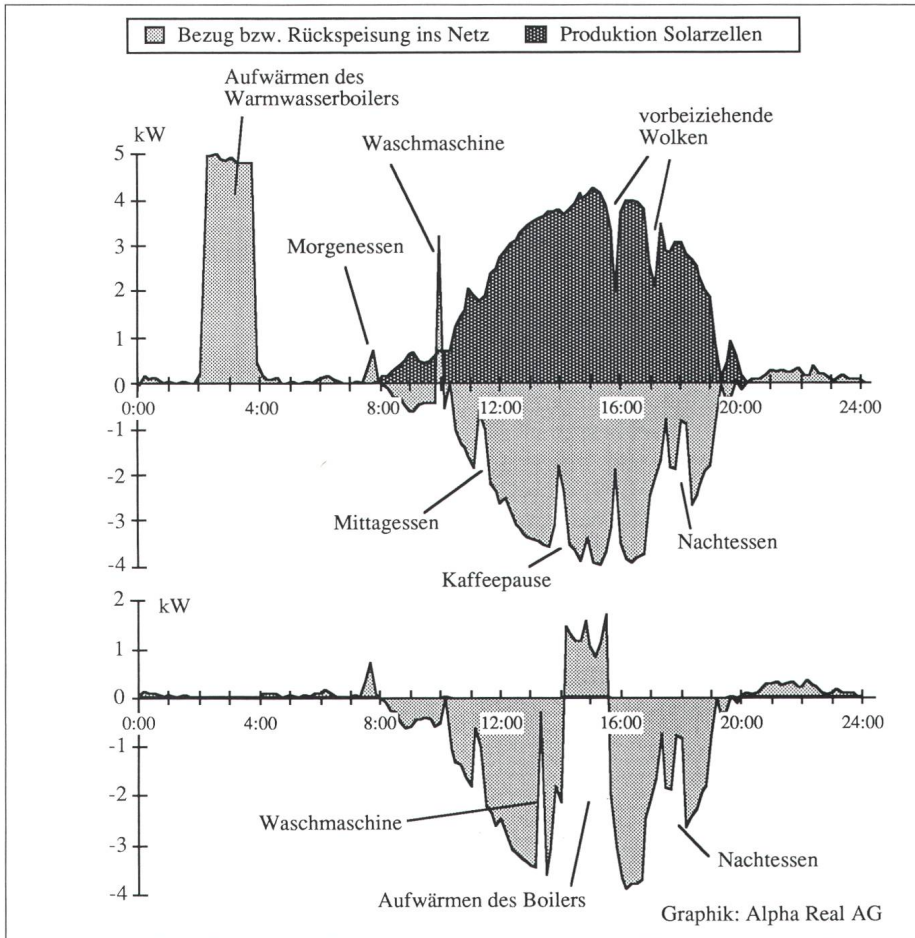
Figur 5 Simulierte Lastverschiebung an einem sonnigen Tag (24. April 1989). Das Diagramm oben zeigt die gemessenen Tagesverläufe von Produktion (■) sowie der Summe von Produktion und Verbrauch (■) der Netzbelastung. Das untere Diagramm zeigt die reduzierte Netzbelastung bei Verlegen der Boilererwärmung in die Zeit der maximalen Produktion. Bei der Solarzellenanlage Mönchaltorf liegt dieses Maximum im frühen Nachmittag, weil die Zellen relativ stark gegen Westen orientiert sind. Je weniger die Solarzellenanlage dann produziert, desto stärker würde die Netzbelastung durch die Boilererwärmung.
