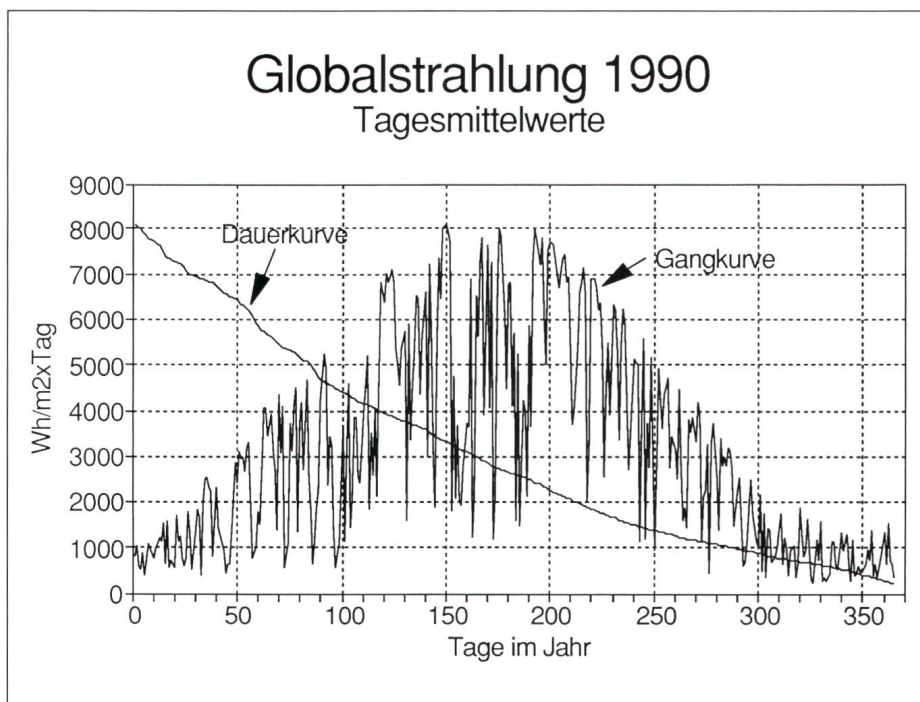
Bild 2 Globalstrahlung 1990, Tagesmittelwerte
