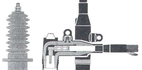
STECKERSYSTEM-SERIE 200 Bis max. 24 kV - 250 Amp.
