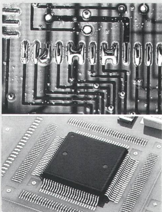
Verschiedene Lötsergebnisse
