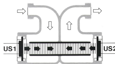
Durchfluß-Messung mit Ultraschallsonden US1 und US2
