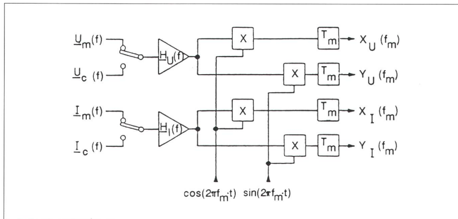
Figure 9 Schéma des circuits d'entrée
