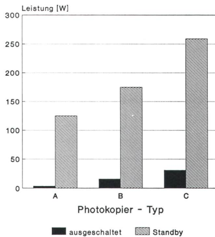
Bild 9 Leistungsaufnahme verschiedener Fotokopiertypen im Standby-Betrieb und ausgeschaltet
