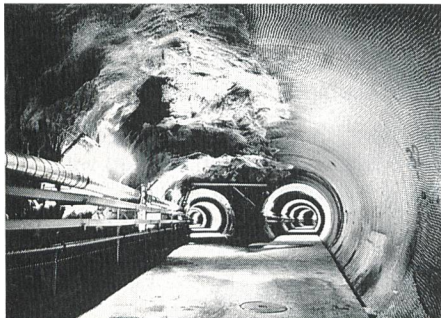
Stollenverzweigung im Nagra-Felslabor auf der Grimsel Galeries du laboratoire souterrain de la Cédra au Grimsel
