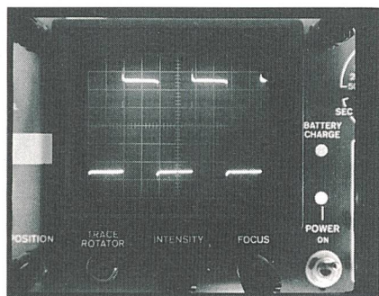
Bild 10 Ausgangsspannung im Leerlauf (Wechselrichter Typ C)
