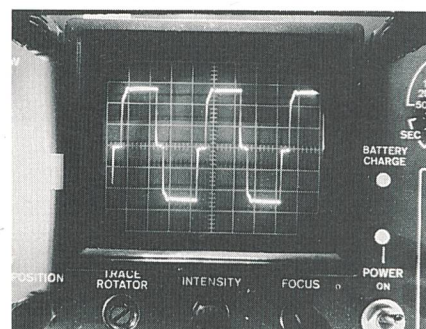
Bild 14 Ausgangsspannung bei Vollast (Wechselrichter Typ D)
