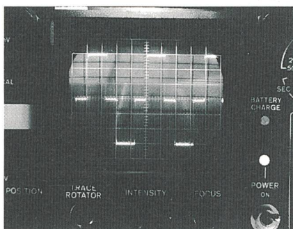
Bild 13 Ausgangsspannung bei Teillast (Wechselrichter Typ D)
