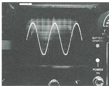
Bild 7 Ausgangsspannung bei Vollast (Wechselrichter Typ A)
