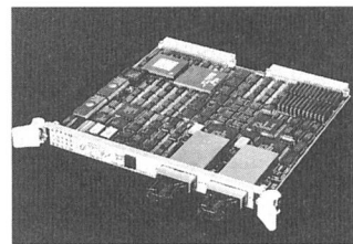
FDDI-Netzwerkkarte
