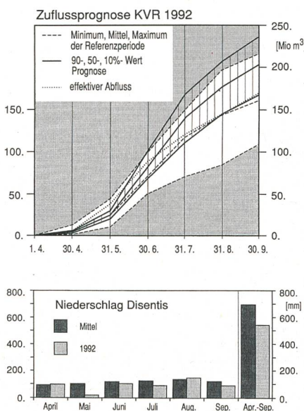
Bild 2. Langfristprognose (Saisonprognose) des kumulierten Zuflusses zur Speicherstufe der Kraftwerke Vorderrhein AG (KVR), ausgegeben am 3. April 1992. Die gestrichelte Fläche beinhaltet die Spanne, in der sich mit 80% Wahrscheinlichkeit der kumulierte Abfluss bewegen wird (Prognoseintervall). Wie die untere Darstellung zeigt, war wegen eines im Vergleich zum klimatologischen Wert zu trockenen Sommers 1992 der kumulierte Zufluss Ende September am unteren Rand des Prognoseintervalls
