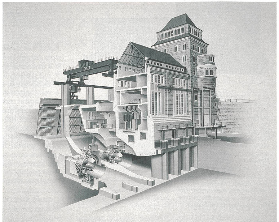
Bild 1 Schnitt durch das Kraftwerk Laufenburg. Durch Modernisierung und den Einbau neuer Turbinen/Generatoren ist die jährliche Produktion um über 100 Gigawattstunden gesteigert worden
