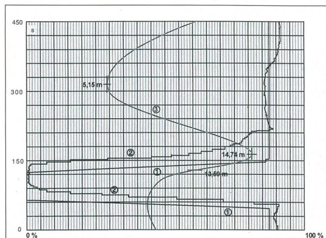
Kurve 1: Sollwertvorgabe Kurve 2: die vom Rechner gefahrenen Kraftwerksleistung Kurve 3: Wasserschlossschwingung. Diese Kurve wurde während der Optimierung der dynamischen Bewertung aufgenommen, wo mit simuliertem Seepiegel (siehe entspr. Abschnitt) gefahren wurde, um bei etwaigen «Ausreissern» die Anlage nicht zu gefährden.
