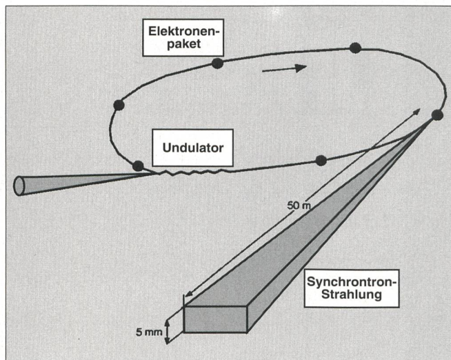
Synchrotronstrahlung: Elektronen, die in einem Speicherring mit hoher Geschwindigkeit zirkulieren, senden eine sehr intensive, stark nach vorn gebündelte elektromagnetische Strahlung aus
