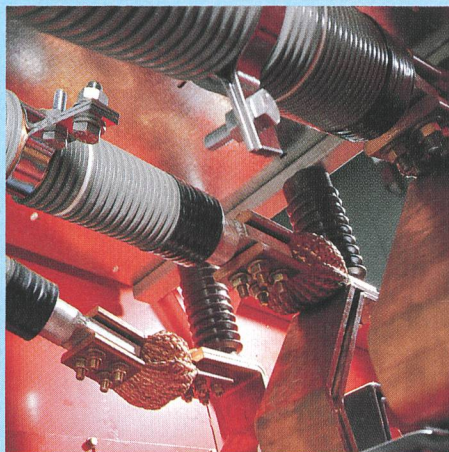
DURESCA®-Stromschiene Typ DE, während der Montage
