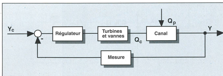
Figure 1 Schéma de principe du réglage du niveau en amont d'un barrage au fil de l'eau
