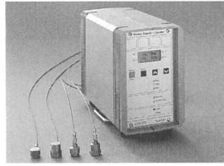
4-Kanal-Kuppler 5134 mit angeschlossenen Sensoren
