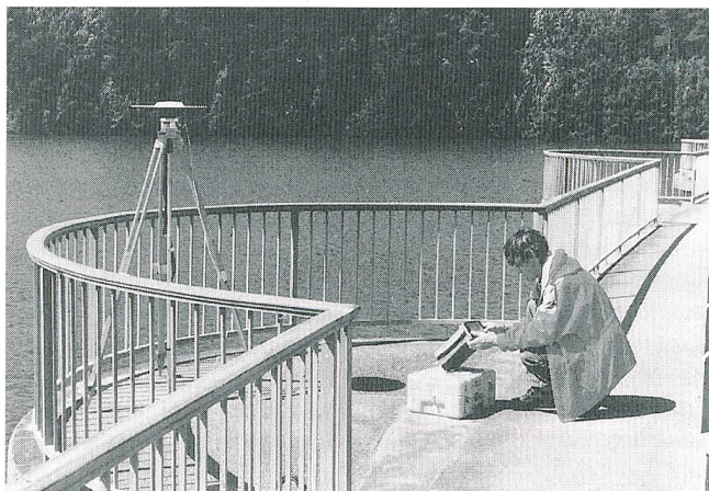
Die Stauwand des Schiffensees (FR) wurde als eine der ersten mit dem auf Satelliten beruhenden «Globalen Positionier-System» (GPS) vermessen. Links die genau positionierte Spezialantenne für den Empfang der Funksignale aus dem Weltraum (Bild: H. Waldschmidt)
