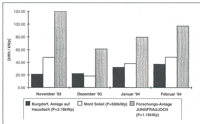
Bild 7 Auf die Anlageleistung bezogene spezifische Energieproduktion der Anlage Gfeller/Burgdorf (3,18 kW_p ), Mont-Soleil (560 kW_p ) und Jungfrauoch (1,152 kW_p ) im November 1993, Dezember 1993, Januar 1994 und Februar 1994
