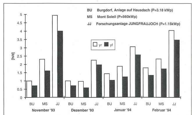
Bild 10 Strahlungsertrag Y_r und Endertrag Y_f bei den Anlagen Gfeller/Burgdorf ( 3,18 \text{ kW}_p ), Mont-Soleil ( 560 \text{ kW}_p ) und Jungfrauoch ( 1,152 \text{ kW}_p ) in den Monaten November 1993, Dezember 1993, Januar 1994 und Februar 1994
