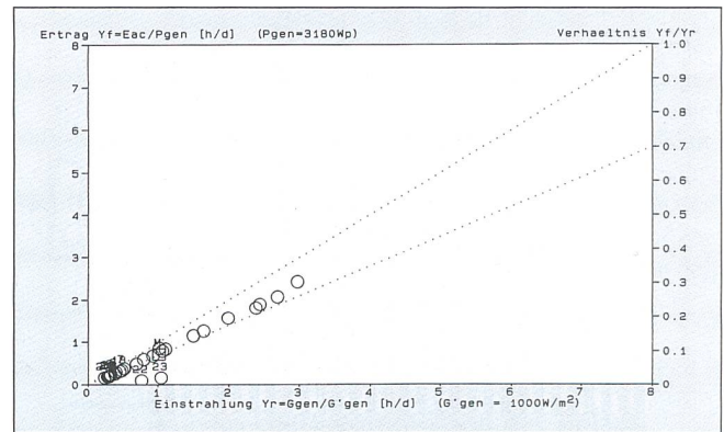
Bild 9 Strahlungsertrag Y_r , Endertrag Y_f und Nutzungsziffer PR = Y_f/Y_r bei der Anlage Gfeller in Burgdorf im November 1993. Am 22. und 23. November 1993 war der Solargenerator mit Schnee bedeckt
