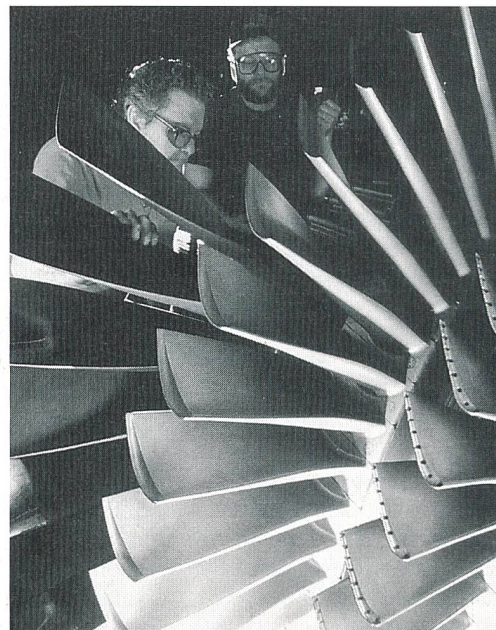
106-MW-Gasturbine von Siemens: Im laufendem Betrieb sind die Schaufeln Verbrennungsgasen bis zu 1400°C ausgesetzt
