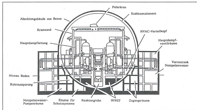
Sphärisches Stahlcontainment des Systems 80+
